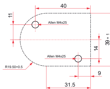
SCHEEM OF FASTENING ESQUEMA DE FIJACIÓN
